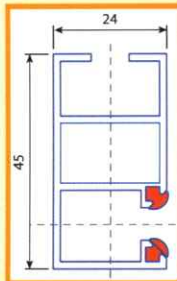
Einfachkasten-FS
