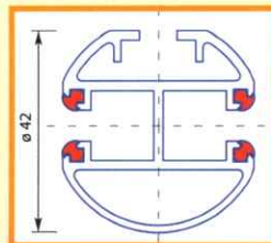
Doppelrund-FS
