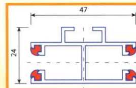
Doppel-FS
