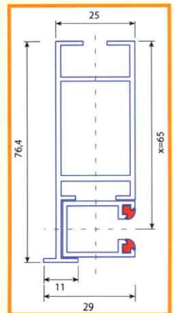
Laibungs-FS (2-Teilig)
