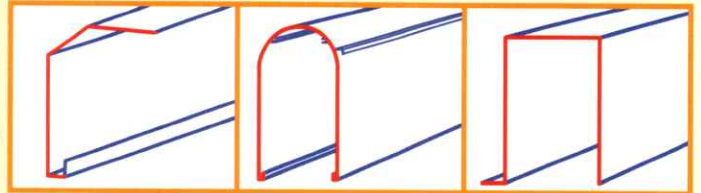
Schrägblende
