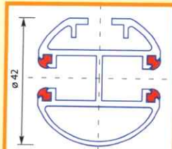
Doppelrund-FS
