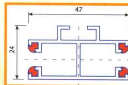
Doppel-FS
