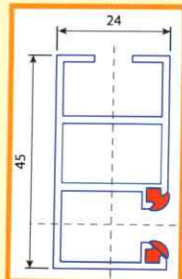
Einfachkasten-FS
