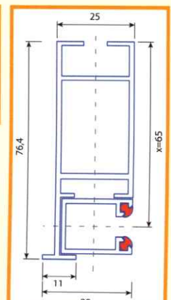
Laibungs-FS (2-Teilig)
