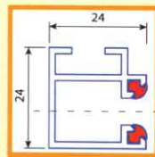
Einfach-FS
